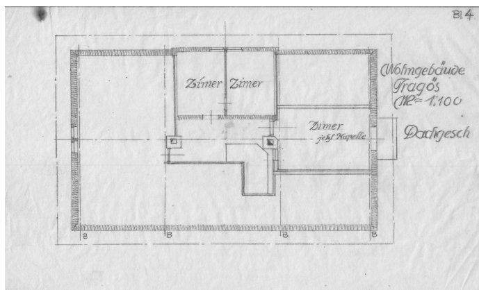
Domūs Tragoessianae ichnographia tabulati subtegulanei.
