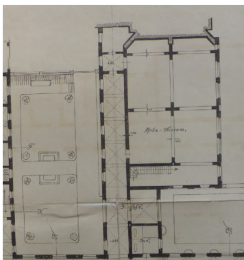
Novi musei ichnographia pedeplanorum.
