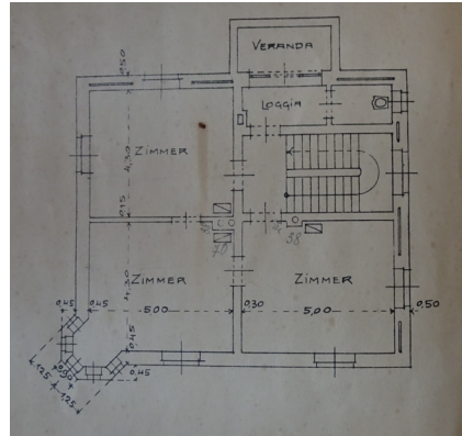
Villae Ottiliensis ichnographiae pedeplanorum primi tabulati.
